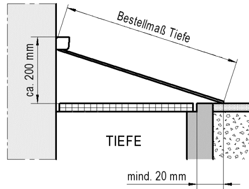
Schnittansicht Tiefe
