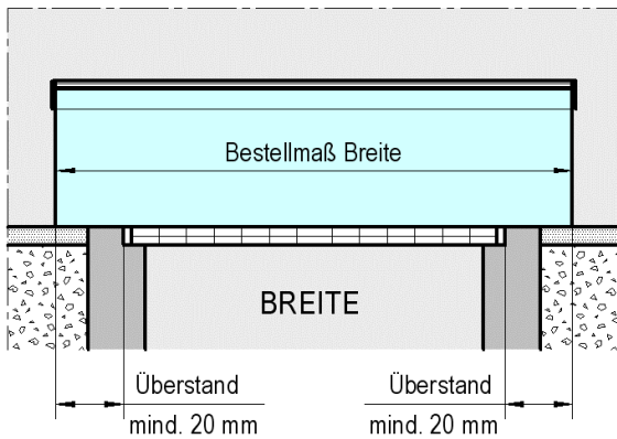
Schnittansicht Breite
