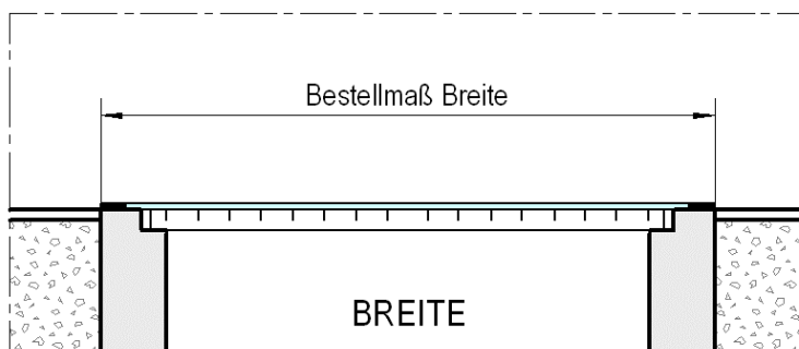
Schnittansicht Breite
