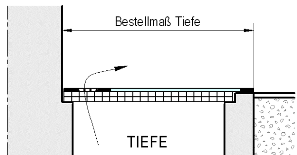
Schnittansicht Tiefe
