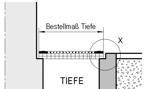
Schnittansicht Tiefe
